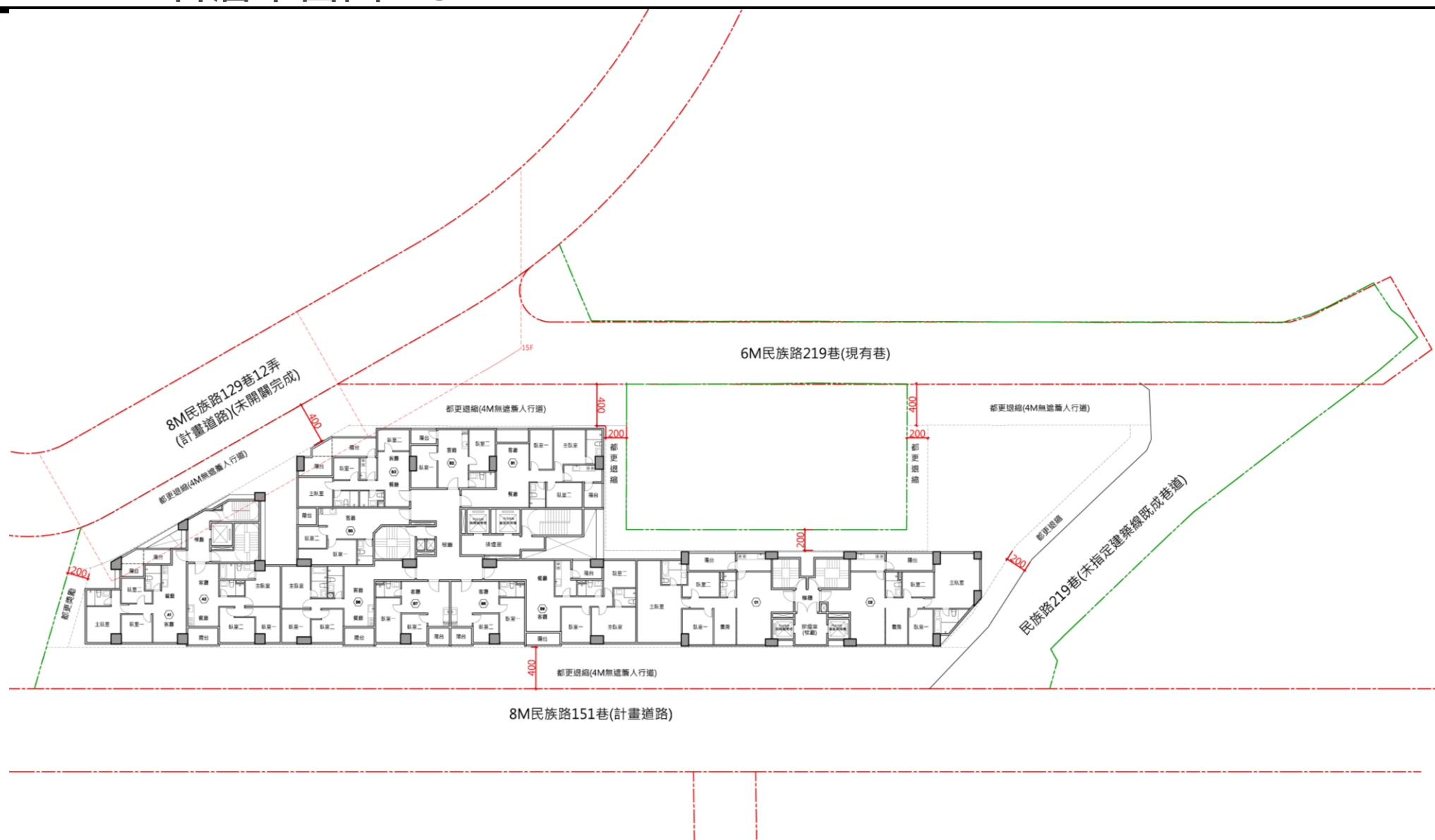
十五層平面圖
