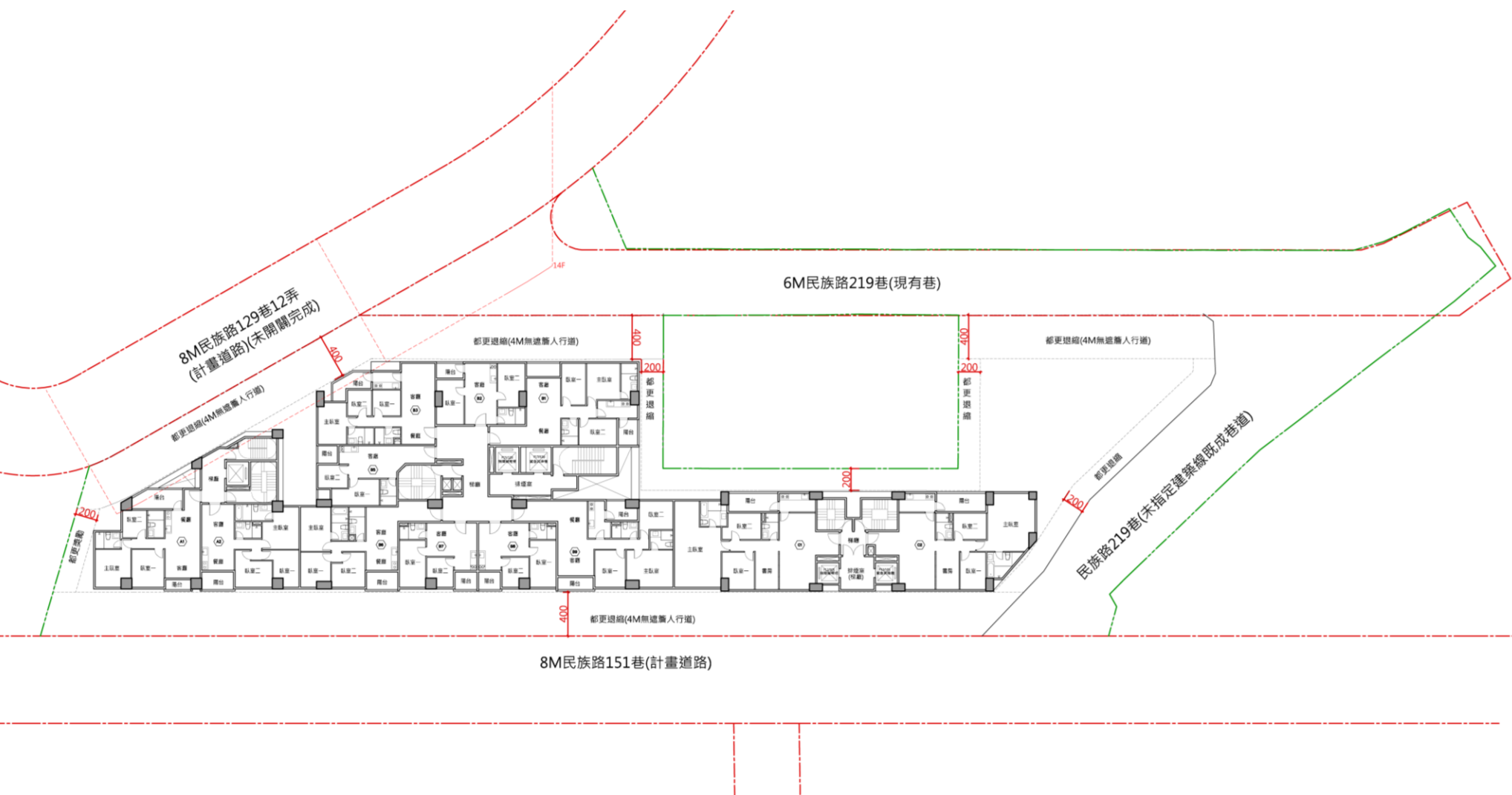
十四層平面圖
