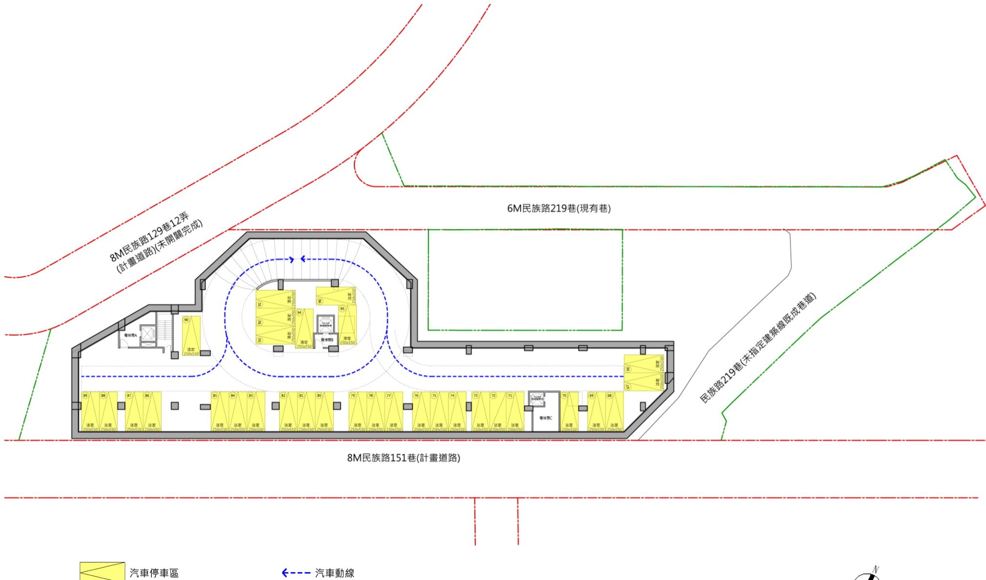
地下三層平面圖
